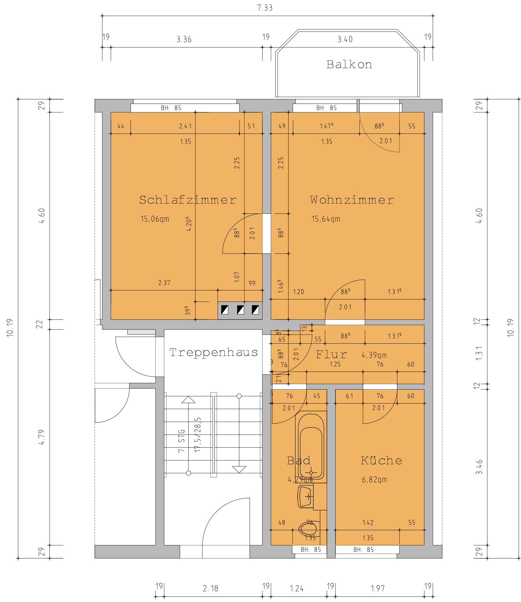
Grundriß Wohnung D – EG bis 3.OG, M 1:50
